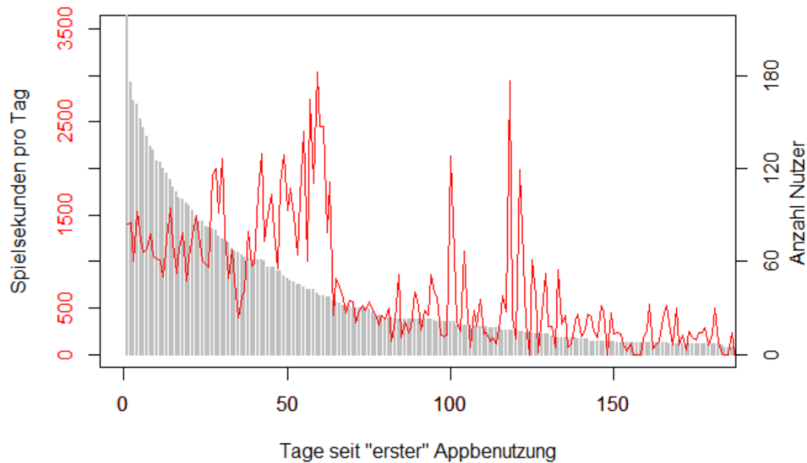
Spieldauer Candy Crush Saga
